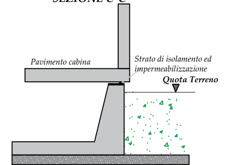
PARTICOLARE SEZIONE C-C
