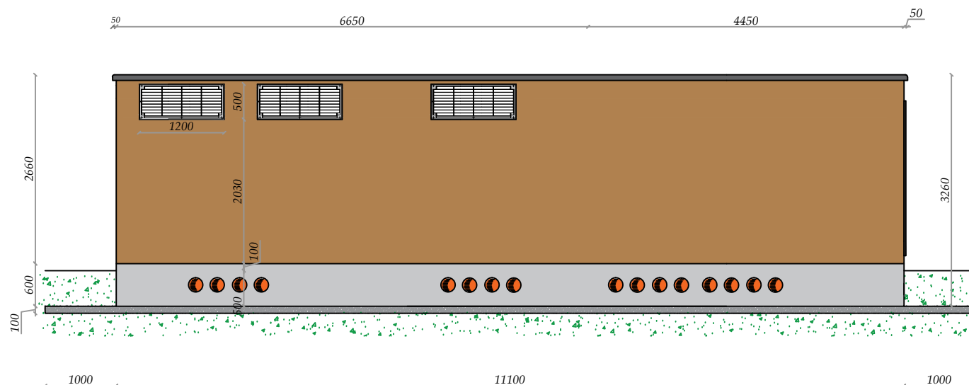
PROSPETTO POSTERIORE
