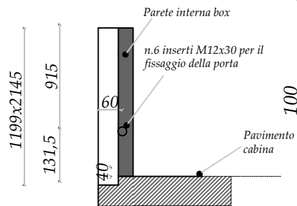
PARTICOLARE SEZIONE A-A
