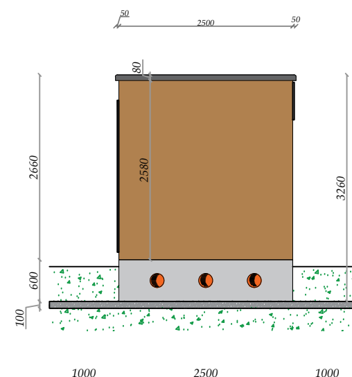
PROSPETTO DX
