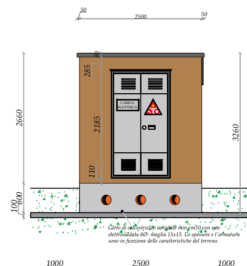
PROSPETTO SX
