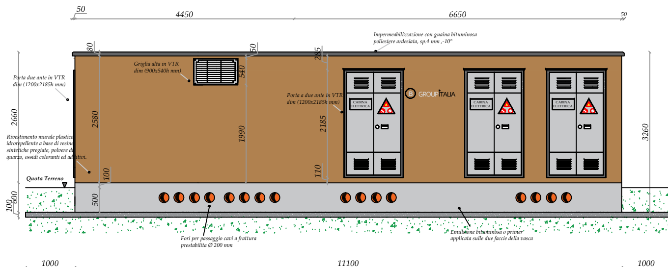
PROSPETTO ANTERIORE
