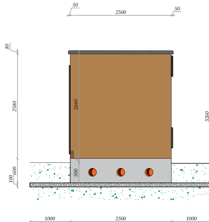
PROSPETTO DX
