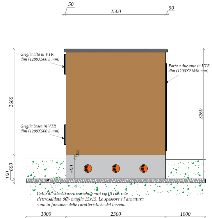
PROSPETTO SX
