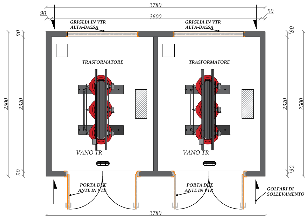
PIANTA
