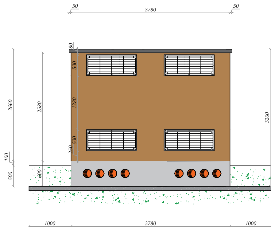
PROSPETTO POSTERIORE
