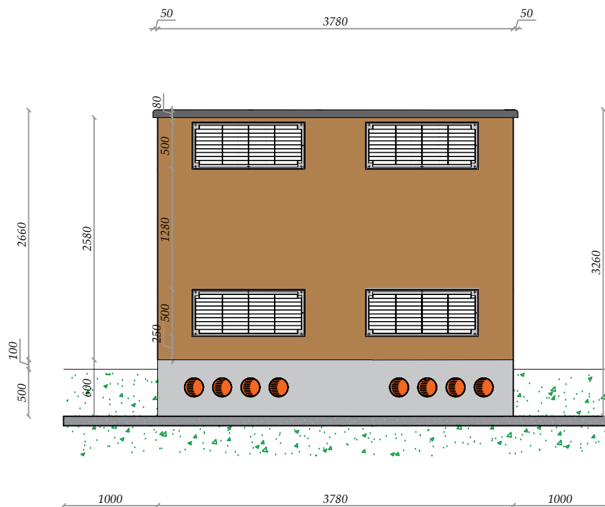
PROSPETTO POSTERIORE
