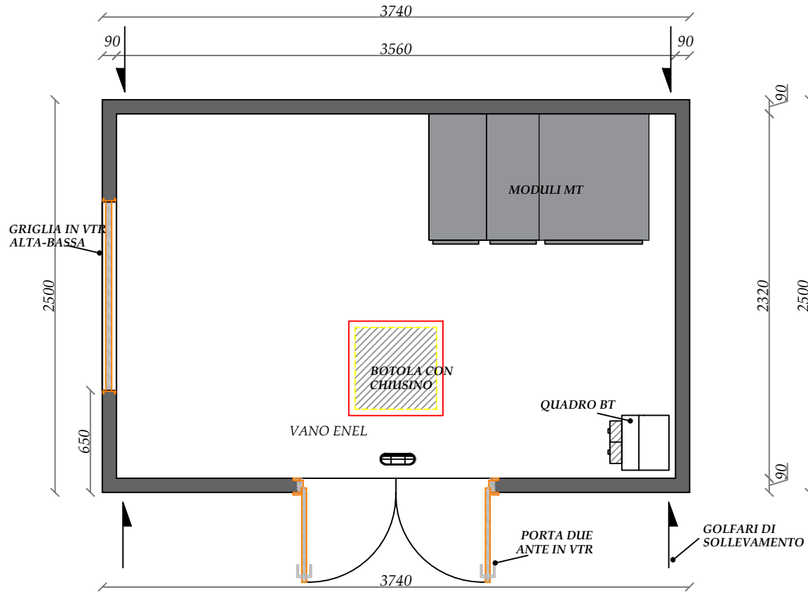
PIANTA
