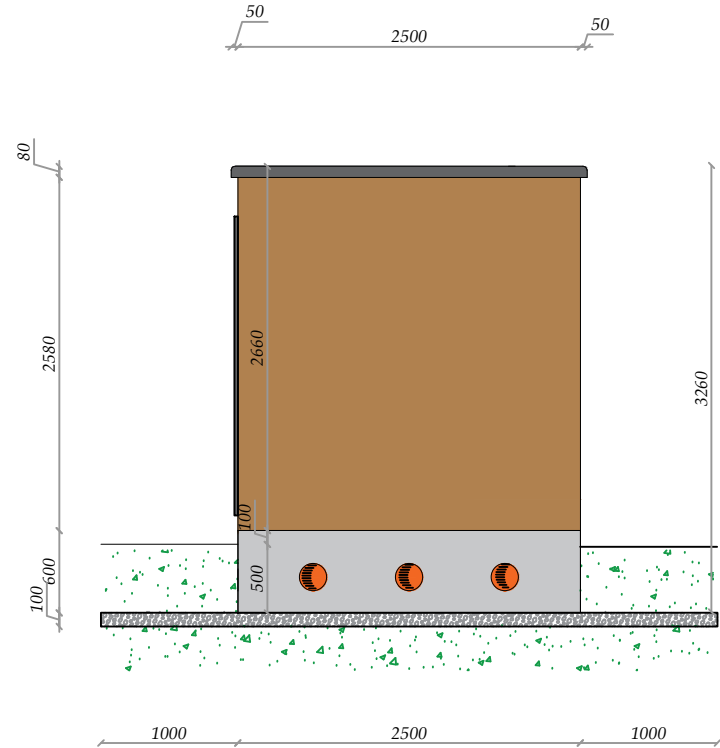
PROSPETTO DX
