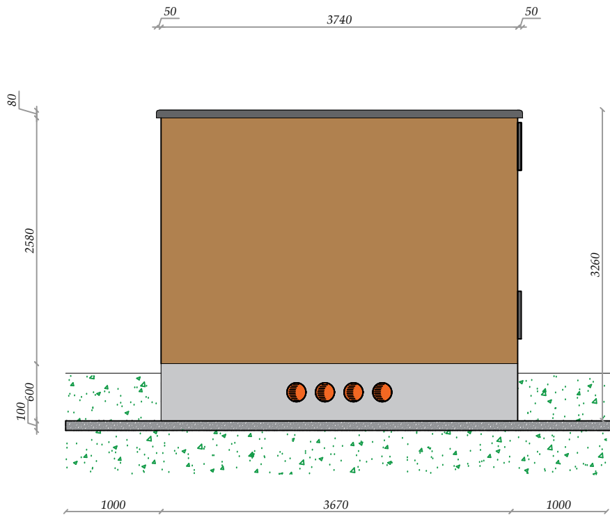
PROSPETTO POSTERIORE
