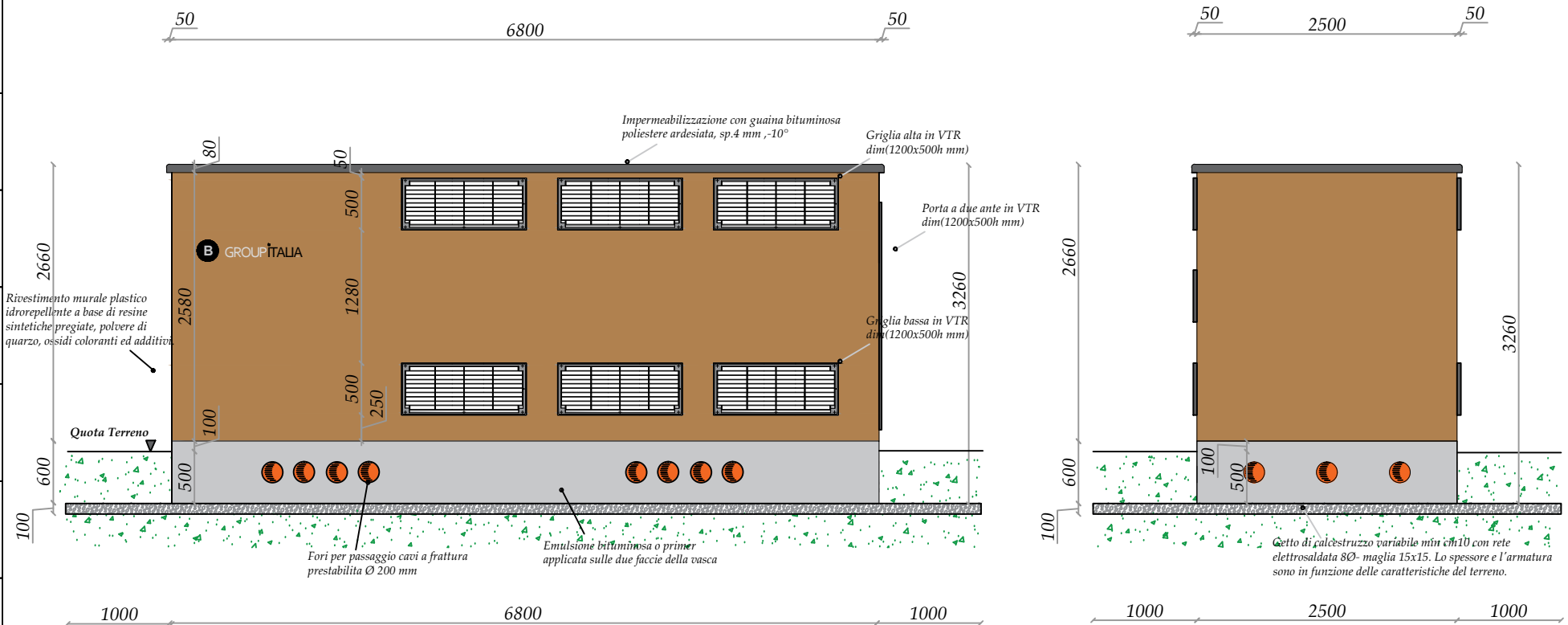
PROSPETTO ANTERIORE
