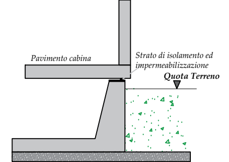
PARTICOLARE SEZIONE D-D
