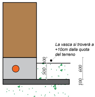
PARTICOLARE VASCA
