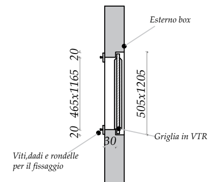
PARTICOLARE SEZIONE B-B
