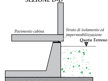
PARTICOLARE SEZIONE D-D
